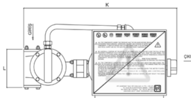
Şekil 2. Sayaç Üstten Görünüşü
