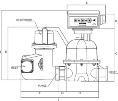
Şekil 1. Sayaç Önden Görünüşü
