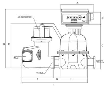
Şekil 1. Sayaç Önden Görünüşü
