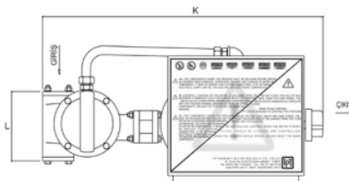
Şekil 2. Sayaç Üstten Görünüşü
