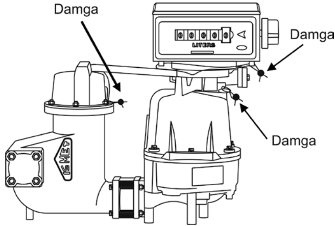
Şekil 12. Damgalama Gösterimi
