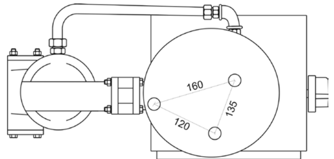
Şekil 3. Sayaç Altın Görünüşü
