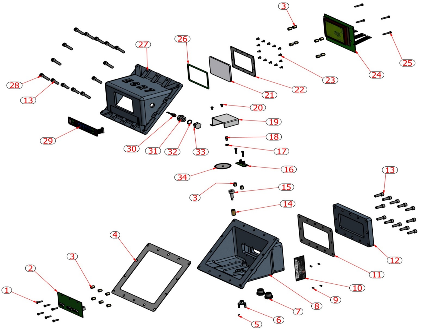
Şekil 16. Elektronik Numaratör Patlamış Resmi
