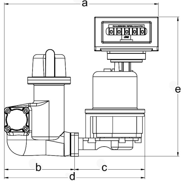
Şekil 2. Sayaç Önden Görünüşü
