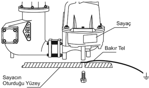
Şekil 5. Topraklama Bağlantısı
