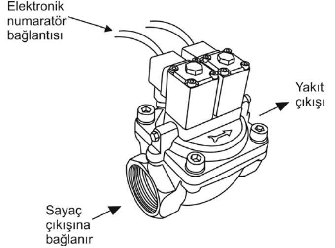
Şekil 4. Solenoid Valf
