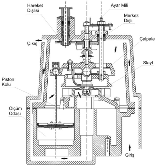
Şekil 6. Çalışma Şekli
