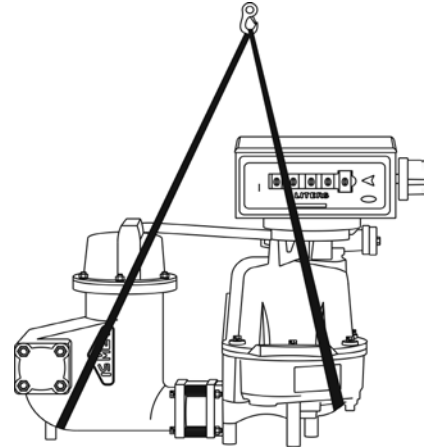
Şekil 11. Sayacın Taşınması
