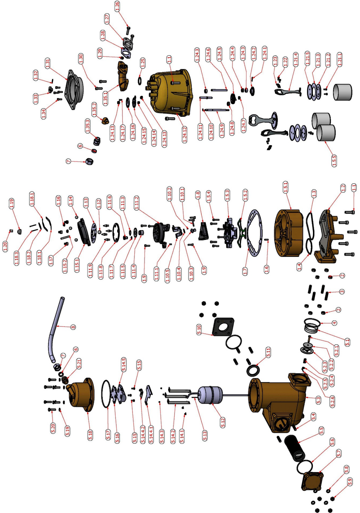
Şekil 15. Sayaç ve Hava Ayırıcı Patlamış Resmi
