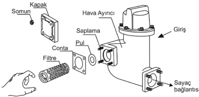
Şekil 14. Hava Ayırıcı Filtrenin Çıkartılması
