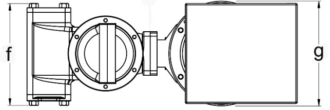
Şekil 1. Sayaç Üstten Görünüşü
