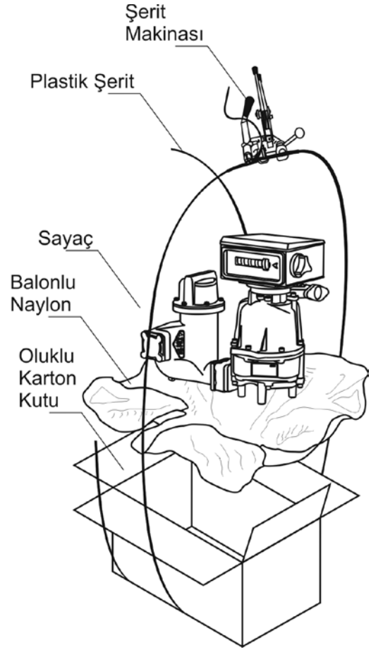
Şekil 10. Ambalajlama Şekli
