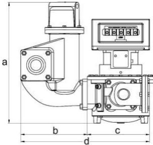
Şekil 1. Sayaç Önden Görünüşü
