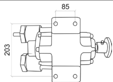
Şekil 3. Pompa Alttan Görünüşü
