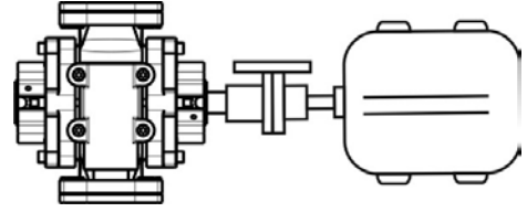
Şekil 7a. Doğru Hizalama – Üstten Görünüş
