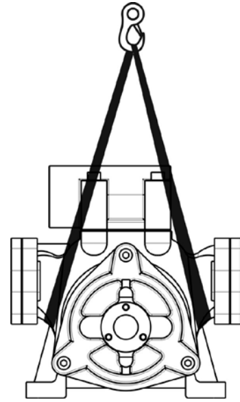
Şekil 15. Pompanın Taşınması
