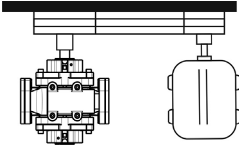
Şekil 9. Doğru Hizalama – Üstten Görünüş
