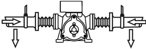
Şekil 10b. Tesisat - Esnek Bağlantı
