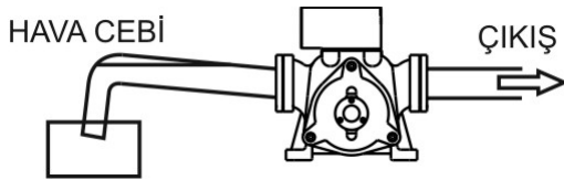
Şekil 10c. Tesisat - Hava Cebi
