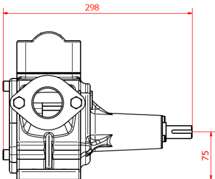
Şekil 2. Pompa Ölçüleri
