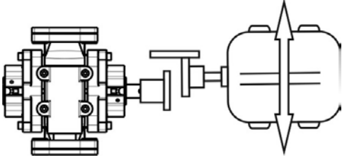
Şekil 6c. Paralel Hizalama – Üstten Görünüş
