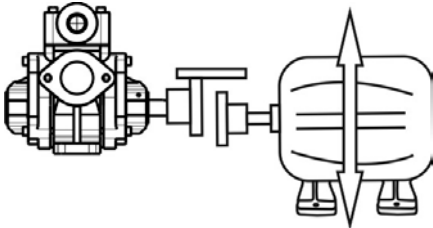
Şekil 6d. Paralel Hizalama – Yandan Görünüş
