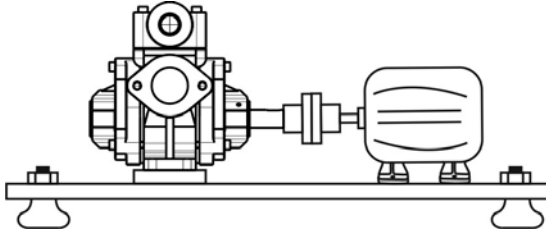
Şekil 5b. Esnek Kurulum
