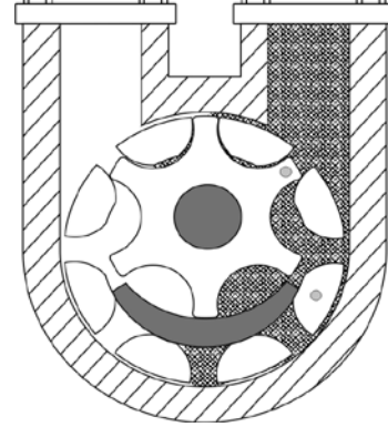
Şekil 13. Çalışma Şekli
