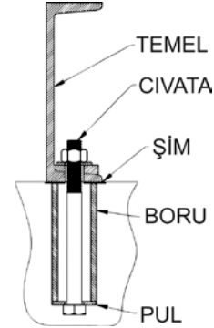
Şekil 4. Ankrajlama
