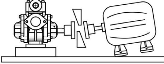
Şekil 6b. Açısal Hizalama – Yandan Görünüş
