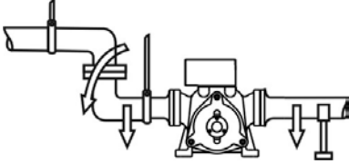
Şekil 10a. Tesisat - Destekler
