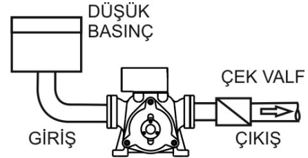
Şekil 10e. Tesisat - Çıkış Çek Valfi
