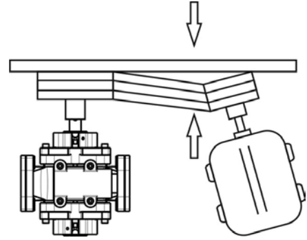
Şekil 8a. Açısal Hizalama – Üstten Görünüş
