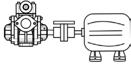
Şekil 7b. Doğru Hizalama – Yandan Görünüş
