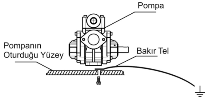
Şekil 12. Topraklama Bağlantısı
