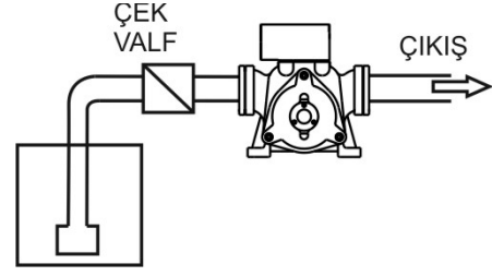
Şekil 10d. Tesisat - Giriş Çek Valfi
