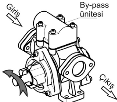
Şekil 11. Pompa Dönüş Yönü
