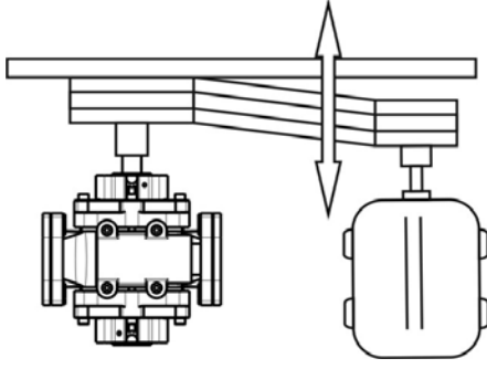
Şekil 8b. Paralel Hizalama – Üstten Görünüş
