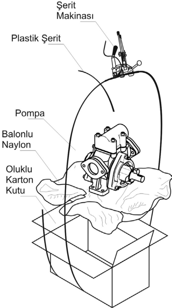
Şekil 14. Ambalajlama Şekli
