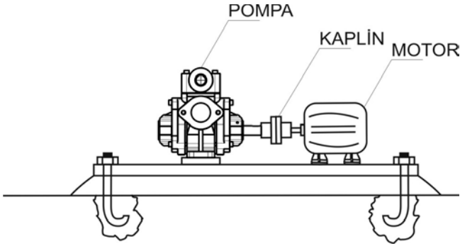
Şekil 5a. Sabit Kurulum
